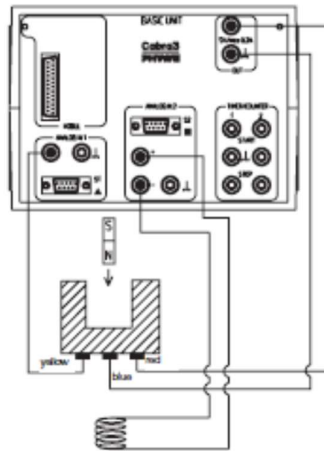
Gambar 2. Diagram rangkaian.
