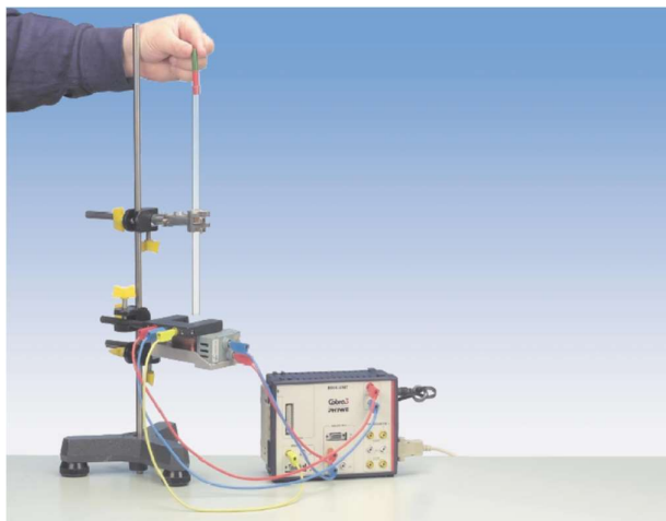
Gambar 1. Rangkaian percobaan impuls induktansi.
