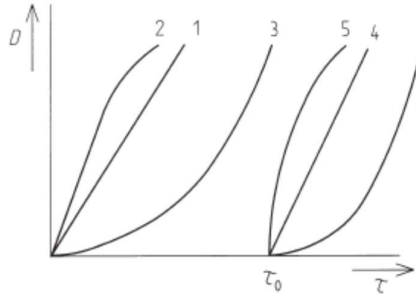
Gambar 1. Gradien kecepatan dan tegangan geser.
